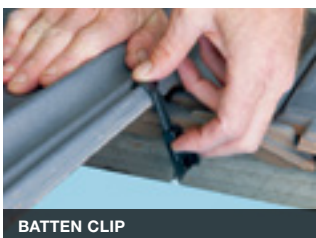
BATTEN CLIP
